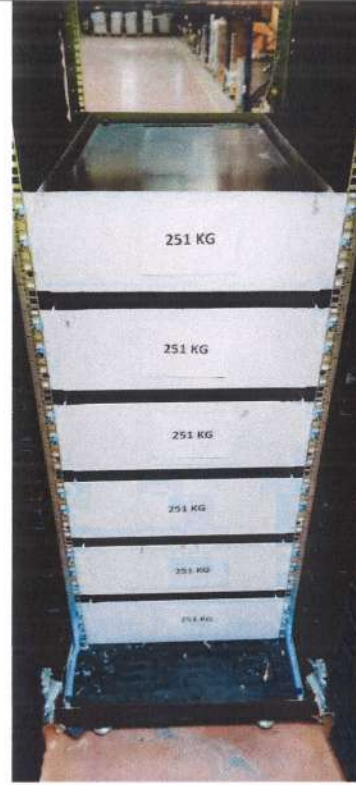
32 U (W=750X,D=1130x H=1666) Cabinet static load test
