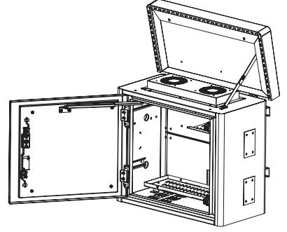
ÖN KAPAK VE ŞAPKA AÇIK İZOMETRİK GÖRÜNÜŞ
