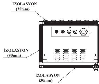
ÜST KESİT GÖRÜNÜŞ
