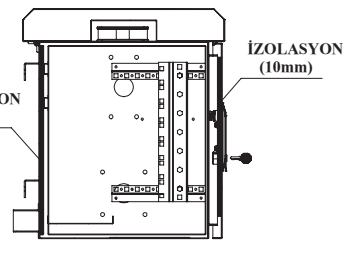
YAN KESİT GÖRÜNÜŞ
