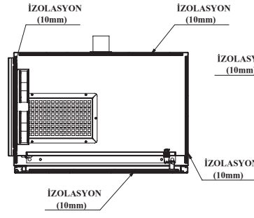
ÜST KESİT GÖRÜNÜŞ
