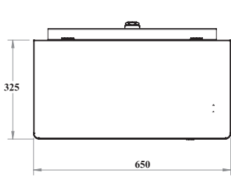
ÜST GÖRÜNÜŞ
