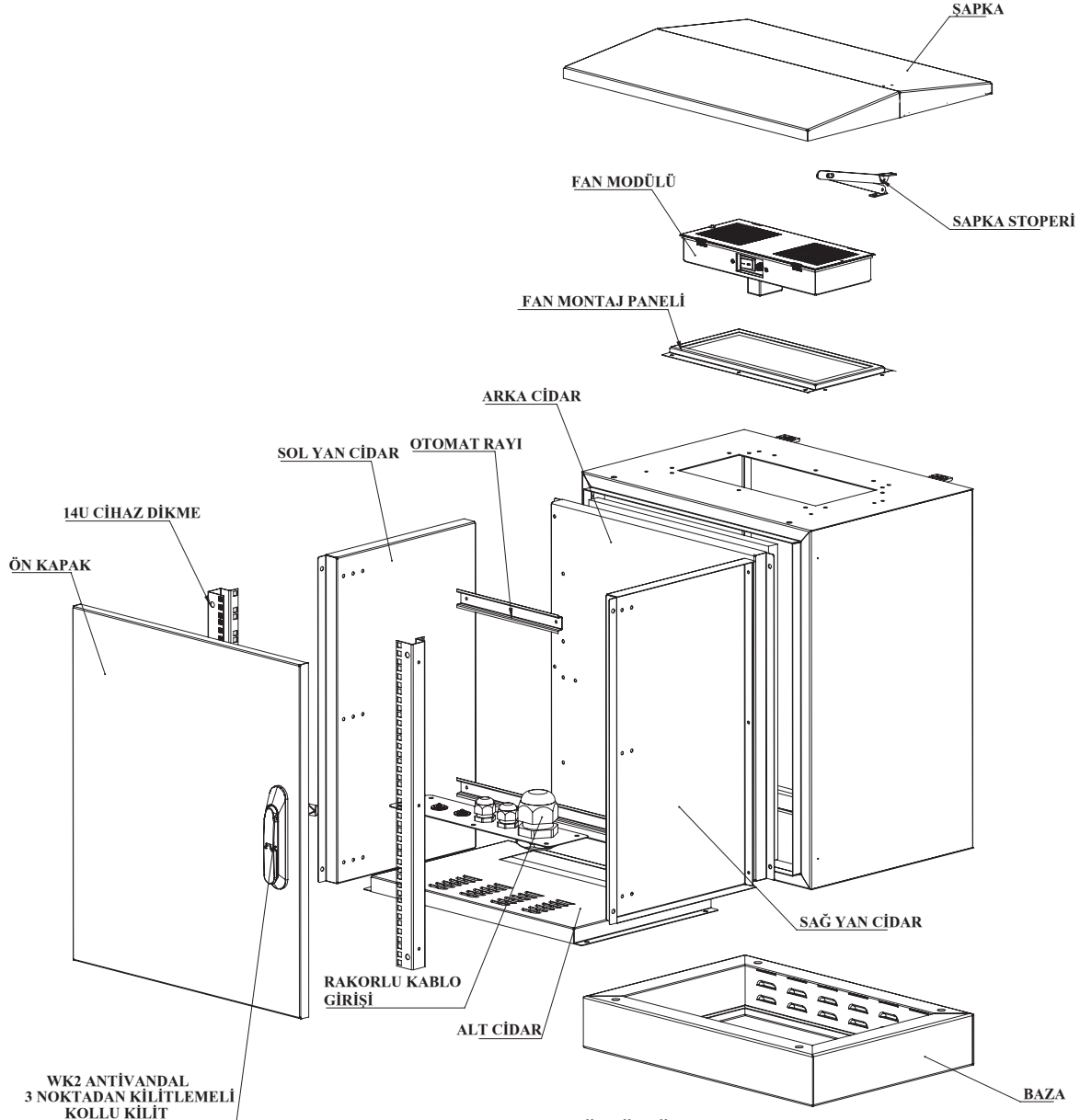
PATLATILMIŞ GÖRÜNÜŞ
