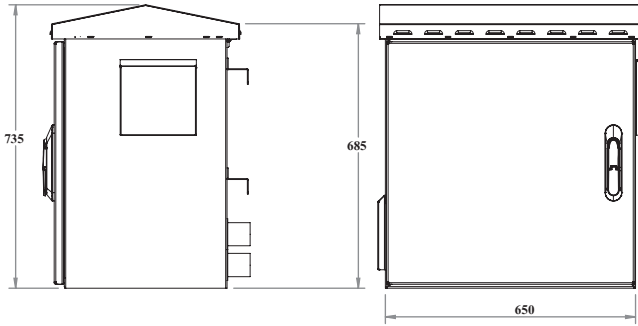
SOL YAN GÖRÜNÜŞ
