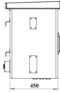
SOL YAN GÖRÜNÜŞ
