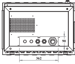
ALT GÖRÜNÜŞ
