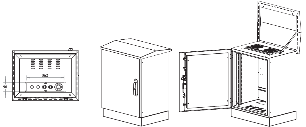
ÖN KAPAK VE ŞAPKA AÇIK İZOMETRİK GÖRÜNÜŞ
