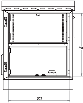
ÖN KAPASIZ GÖRÜNÜŞ
