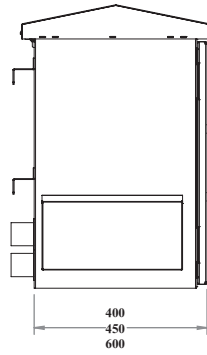
SAĞ YAN GÖRÜNÜŞ
