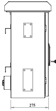
SAĞ YAN GÖRÜNÜŞ
