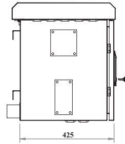
SOL YAN GÖRÜNÜŞ
