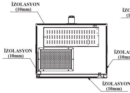
ÜST KESİT GÖRÜNÜŞ
