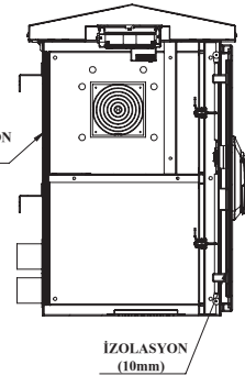
YAN KESİT GÖRÜNÜŞ
