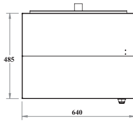
ÜST GÖRÜNÜŞ
