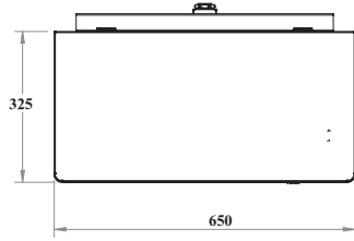
ÜST GÖRÜNÜŞ
