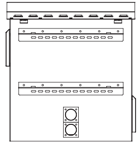
ARKA GÖRÜNÜŞ
