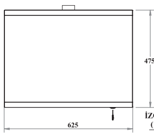
ÜST GÖRÜNÜŞ
