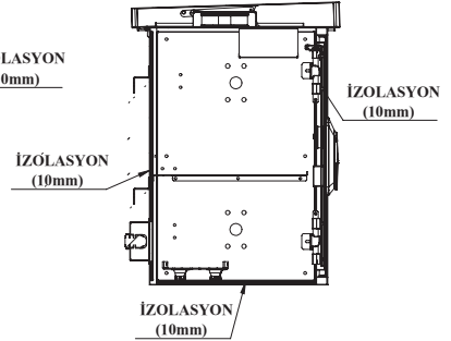
YAN KESİT GÖRÜNÜŞ
