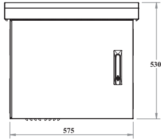
ÖN GÖRÜNÜŞ
