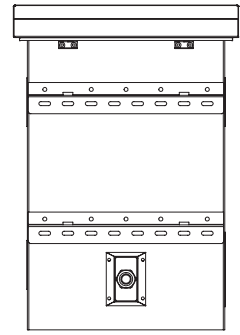
ARKA GÖRÜNÜŞ
