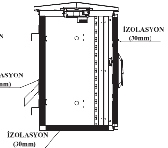
YAN KESİT GÖRÜNÜŞ
