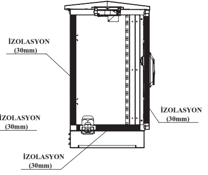
YAN KESİT GÖRÜNÜŞ
