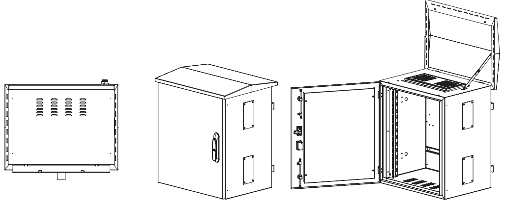
ÖN KAPAK VE ŞAPKA AÇIK İZOMETRİK GÖRÜNÜŞ
