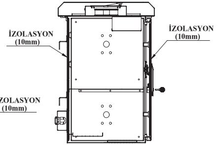
ARKA GÖRÜNÜŞ
