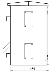
SAĞ YAN GÖRÜNÜŞ
