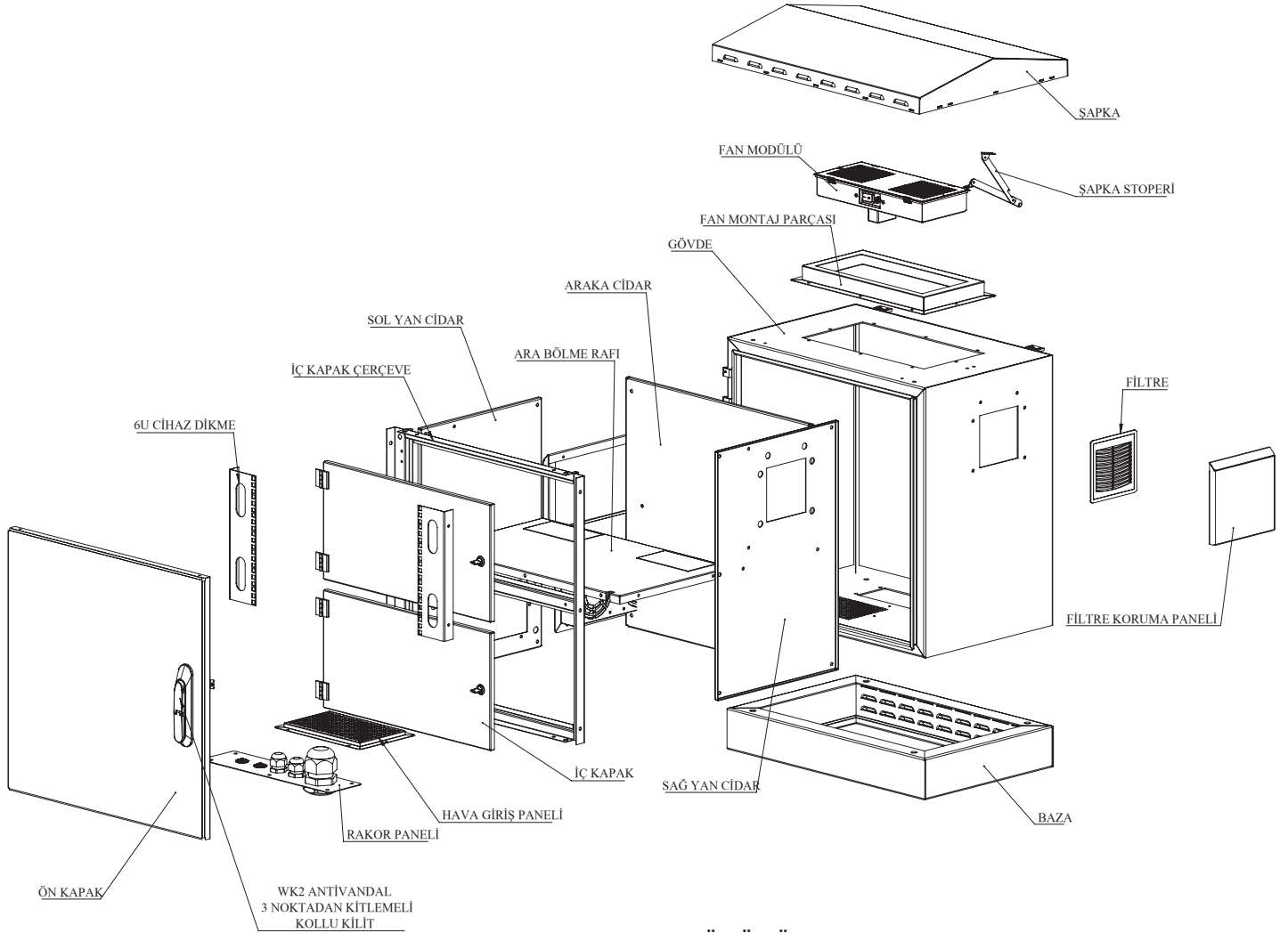
PATLATILMIŞ GÖRÜNÜŞ
