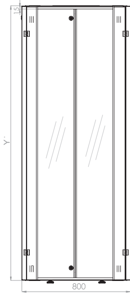
Ön görünüş
