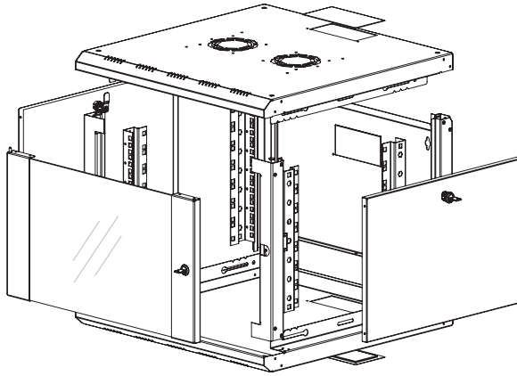
Patlatılmış görünüş
