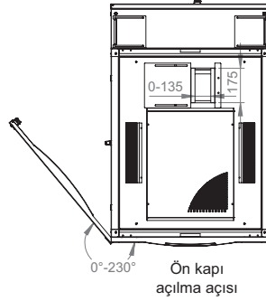
Üst görünüş
