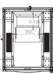
Max/Std/Min Cihaz montaj mesafeleri
