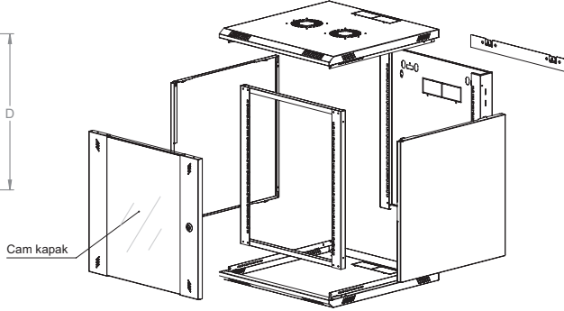
Patlatılmış görünüş
