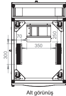
Alt görünüş
