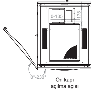
Üst görünüş
