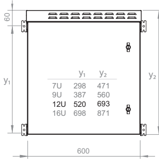
Ön görünüş
