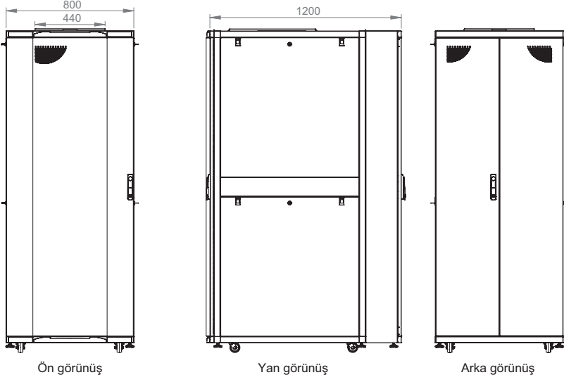
Ön görünüş
