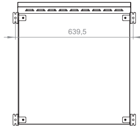
Arka görünüş
