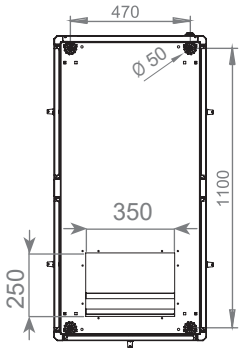
Alt görünüş
