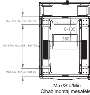
Alt görünüş
