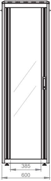
Ön görünüş
