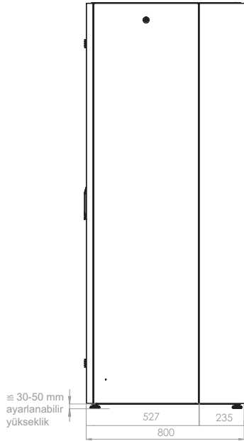
Yan görünüş
