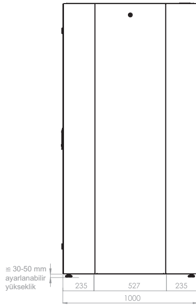
Yan görünüş
