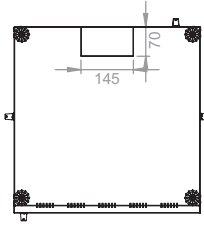
Alt görünüş
