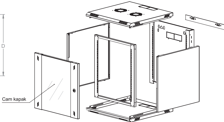
Patlatılmış görünüş
