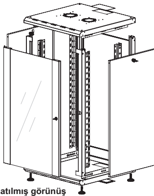
Patlatılmış görünüş
