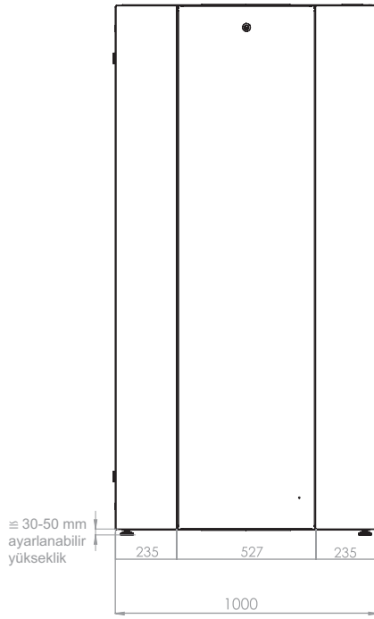
Yan görünüş
