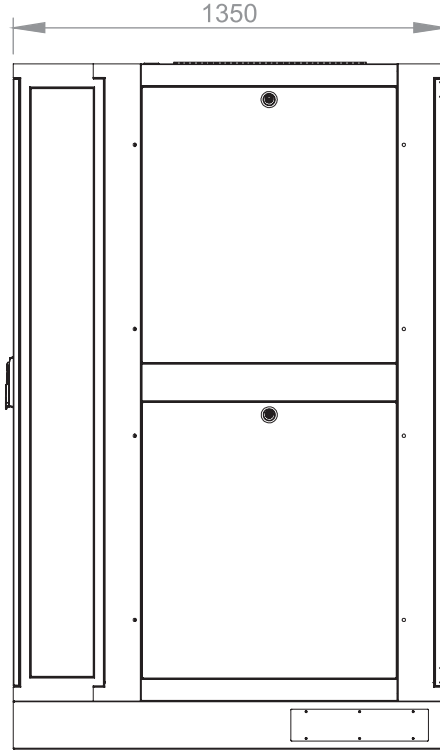
Yan görünüş
