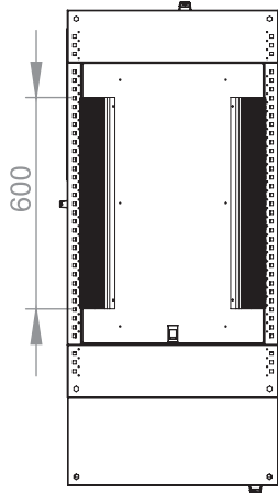
Üst görünüş
